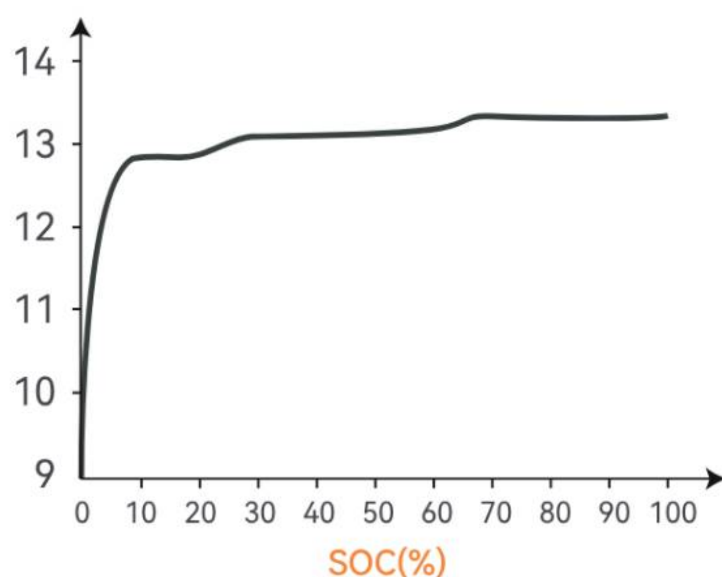
VOLTAGE(V)
